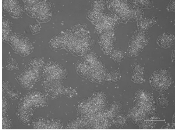
cira-jk-0136-D: passage-3
